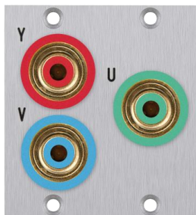
8639646 Worldplate Slot 3 x Cinch YUV Buchse/Buchse
